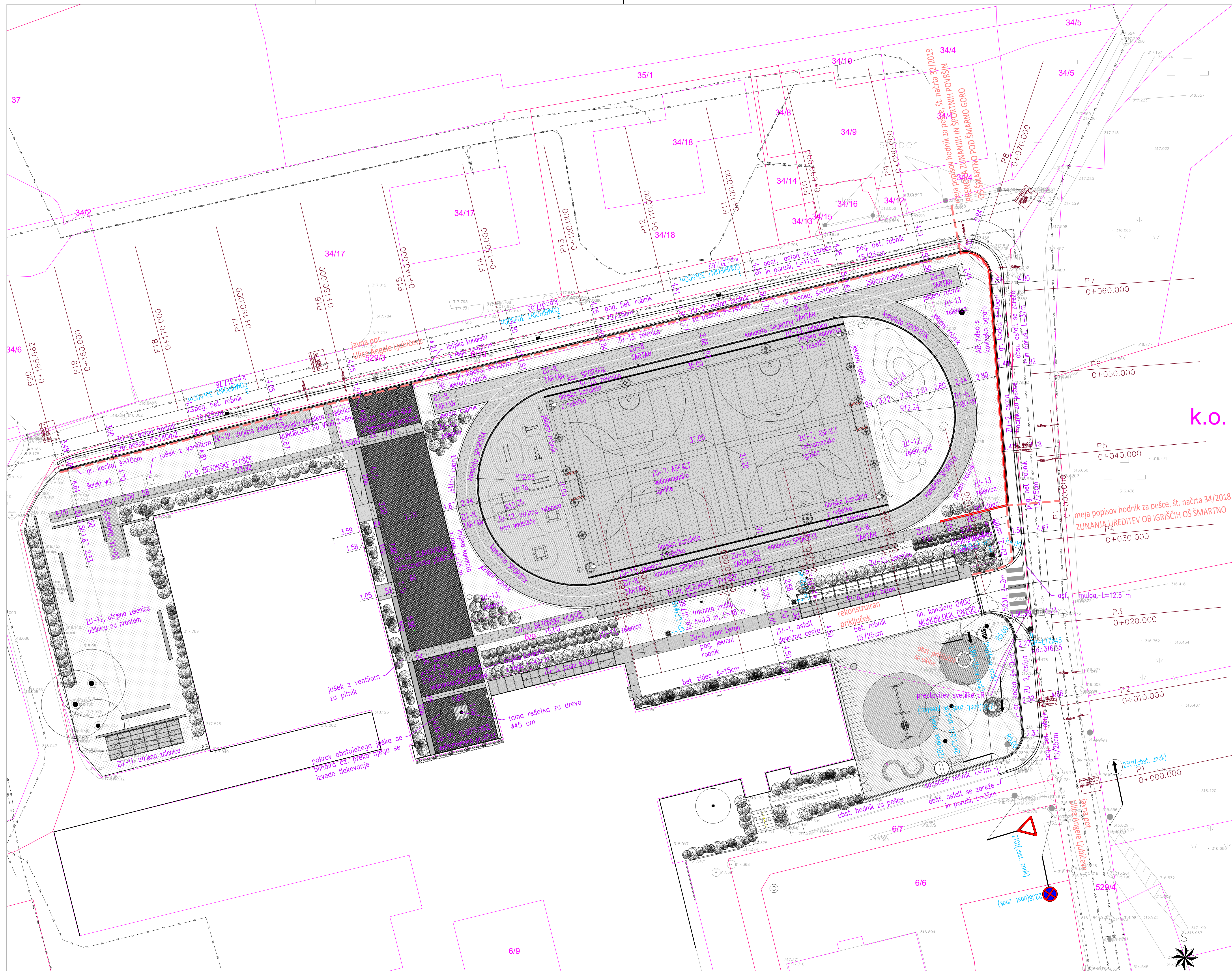
Gradbena situacija M 1:200
